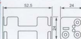
7号 4节 (UM-4*4) Type:A、B
