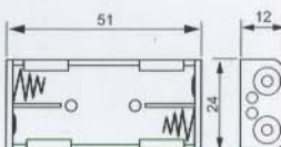
7号 2节 (UM-4*2) Type:A、B
