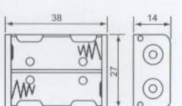
N号 2节 (UM-5*2) Type:A、B
