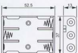
7号 3节 (UM-4*3) Type:A、B、C
